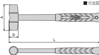
■寸法図
